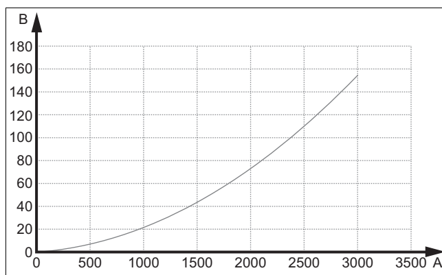
A Debit (l/h) B Pierdere de presiune (kPa)
