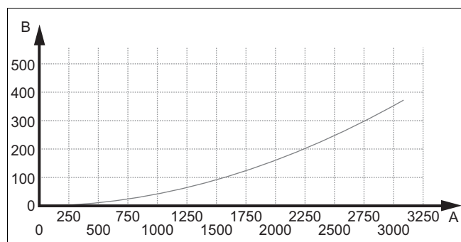
A Debit volumic (l/h) B Pierdere de presiune (mbari)
