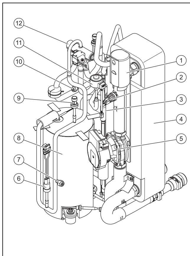
1 Rýchloodvzdušňovač 7 Údržbová prípojka v oblasti vysokého tlaku 2 Snímač tlaku vo vykurovacom okruhu 8 Kompresor 3 Filter 9 Snímač tlaku v oblasti vysokého tlaku 4 Kondenzátor 10 Údržbová prípojka v oblasti nízkeho tlaku 5 Čerpadlo vykurovania 11 Elektronický expanzný ventil 6 Sledovač tlaku v oblasti vysokého tlaku 12 4-cestný prepínací ventil
