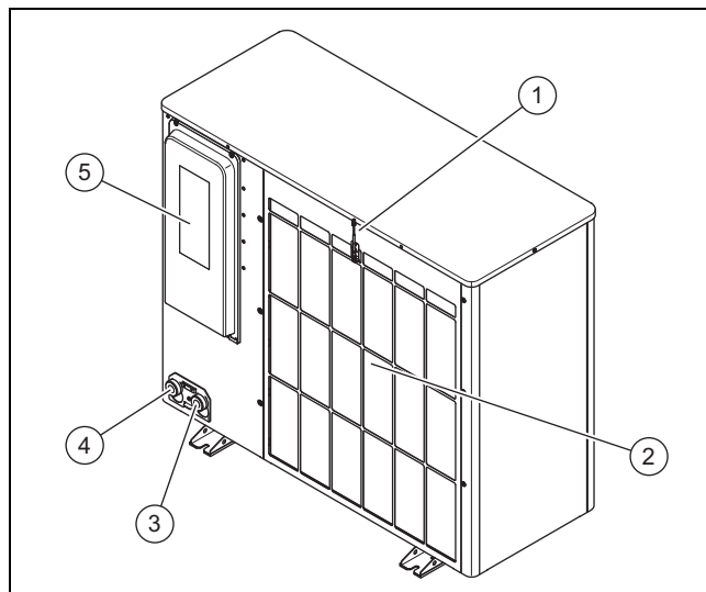
1 Snímač teploty na vstupe vzduchu 4 Prípojka pre spätočku vykurovania, G 1 1/4" 2 Mriežka vstupu vzduchu 5 Kryt elektrických prípojok 3 Prípojka pre výstup vykurovania, G 1 1/4"
