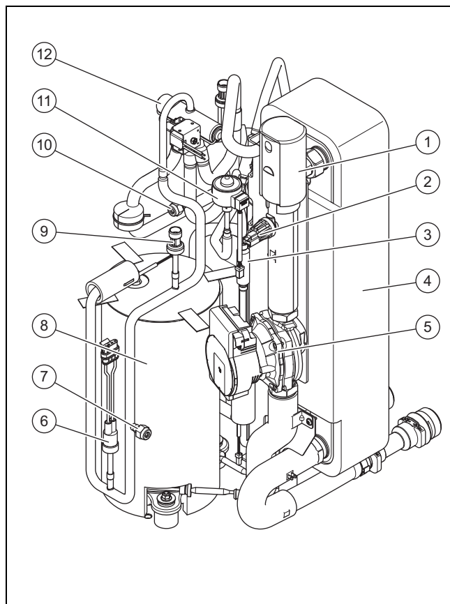
1 Gyors-légtelenítő 6 Nyomásfigyelő a magasnyomású tartományban 2 Nyomásérzékelő a fűtőkörben 7 Karbantartó csatlakozó a magasnyomású tartományban 3 Szűrő 8 Kompresszor 4 Kondenzátor 9 Nyomásérzékelő a magasnyomású tartományban 5 Fűtőköri keringető szivattyú
