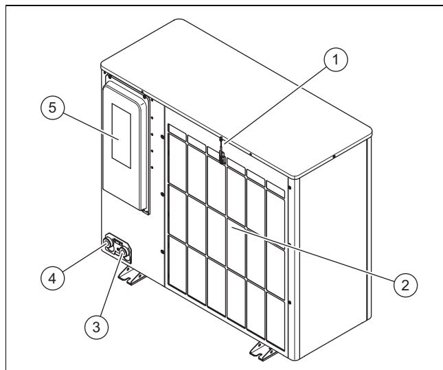
1 Hőmérséklet-érzékelő a levegőbemeneten 4 Fűtési visszatérő ág csatlakozása, G 1 1/4" 2 Levegő belépőbordák 5 Az elektromos csatlakozók burkolata 3 Fűtési előremenő ág csatlakozása, G 1 1/4"
