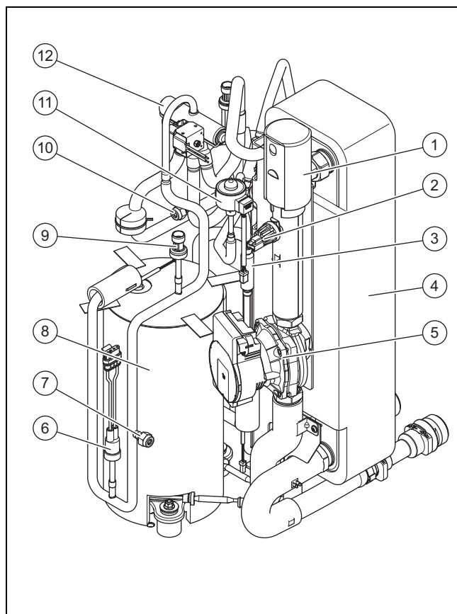
1 Autom. odpowietrznik 6 Czujnik kontrolny ciśnienia w zakresie wysokiego ciśnienia 2 Czujnik ciśnienia w obiegu grzewczym 7 Przyłącze konserwacyjne w zakresie wysokiego ciśnienia 3 Filtr 8 Sprężarka 4 Skraplacz 9 Czujnik ciśnienia w zakresie wysokiego ciśnienia 5 Pompa obiegu grzewczego
